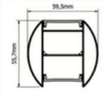
Perfil Embutir 60 x 55 mm *acessórios incluídos
